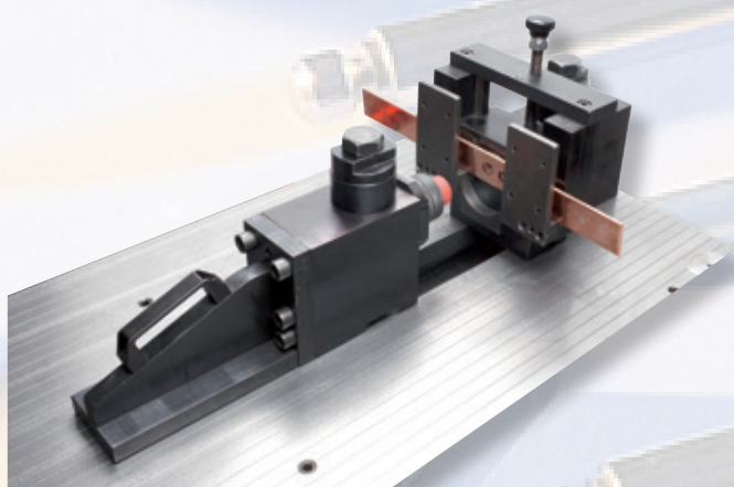
Punzonado barras de distribución Perfuração de barras
