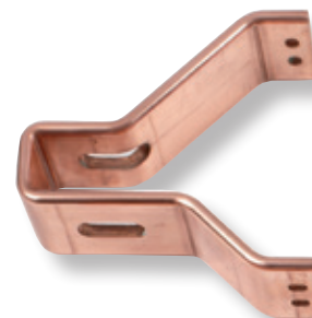
Barra de cobre plegada y punzonada Cuadros eléctricos
