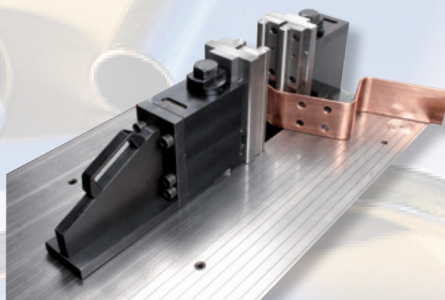
Doblado de barras en U Curvatura do barras em forma de U
