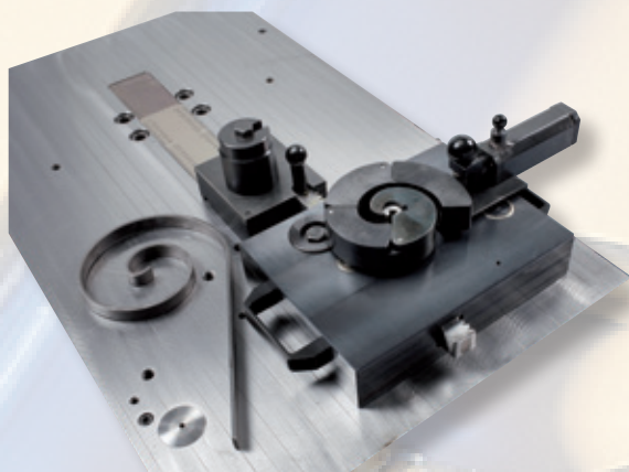
Formación de espirales Formar espirais
